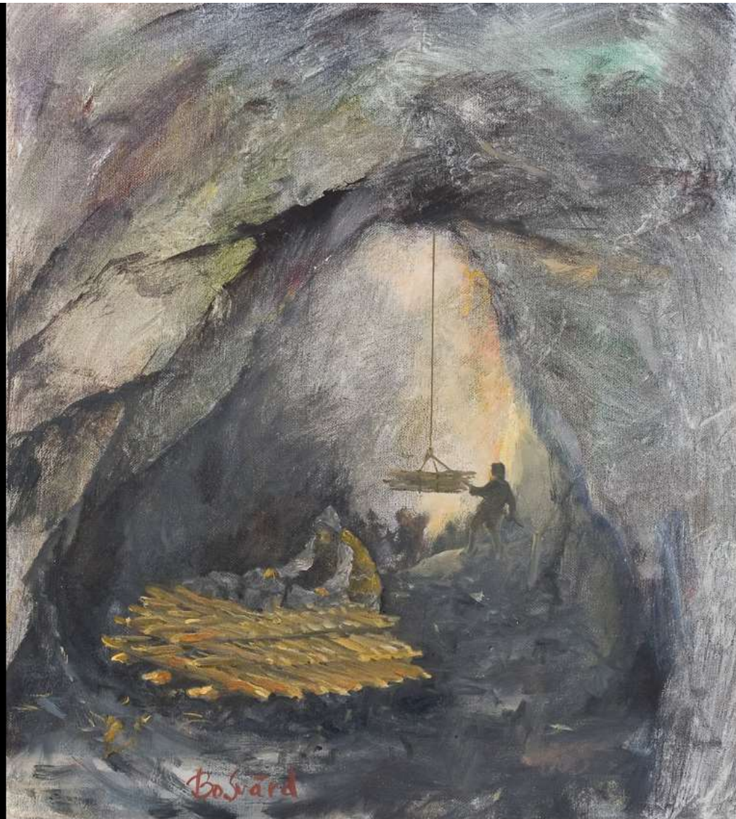
Sänkningslave vid sänkning av schakt. Byggdes något pyramidformad med glesa och täta varv. Överst lades stora stenar för att 'trycka ner' hettan. Veden firades ner i knippen.
