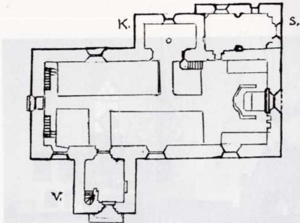
Planskiss över Möklinta kyrka enl uppmätning av ATA
